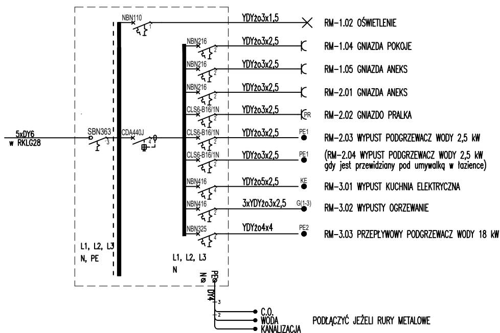
TABLICA RM OBUDOWA WNĘKOWA
